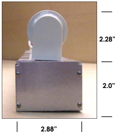
D193WP end view
